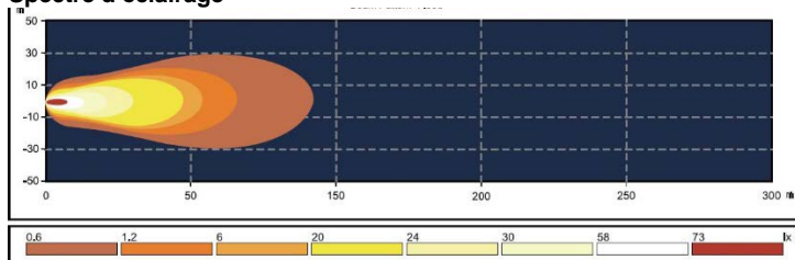
Spectre d'éclairage
